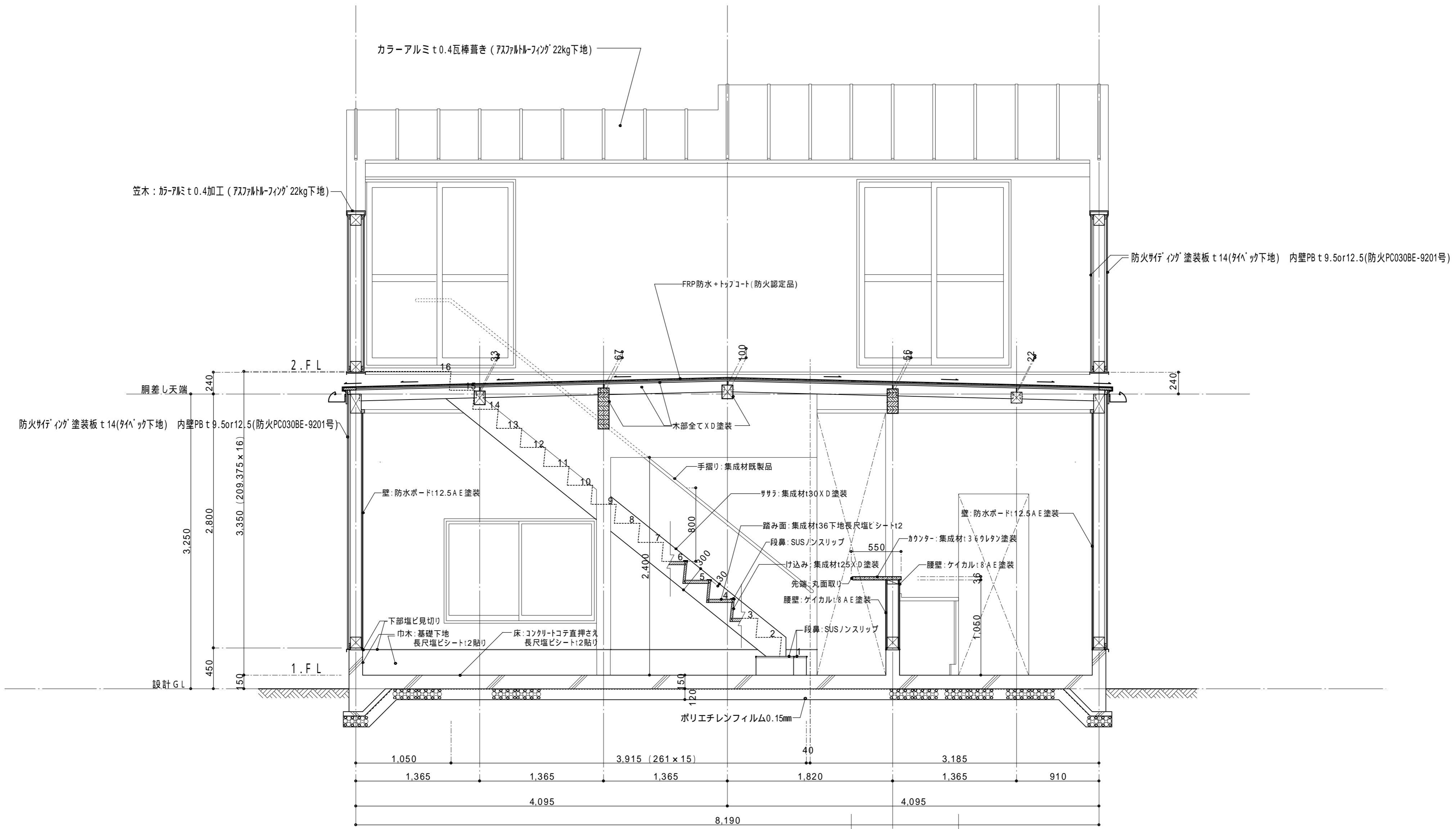
矩計図 - 3 S = 1 / 30
